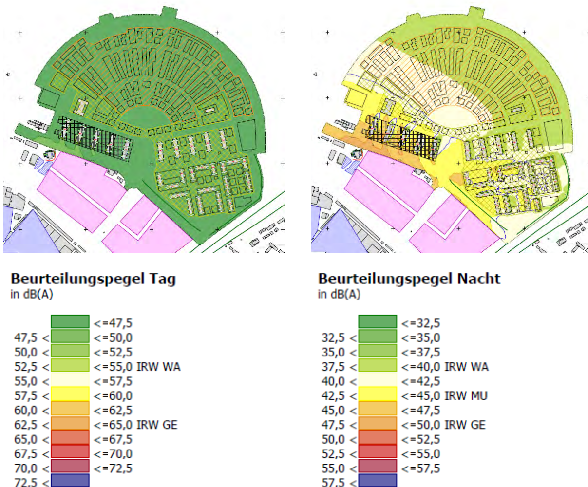
Abb. 34: Gewerbelärm im Plangebiet, Berechnungshöhe 11 m (3. OG)
