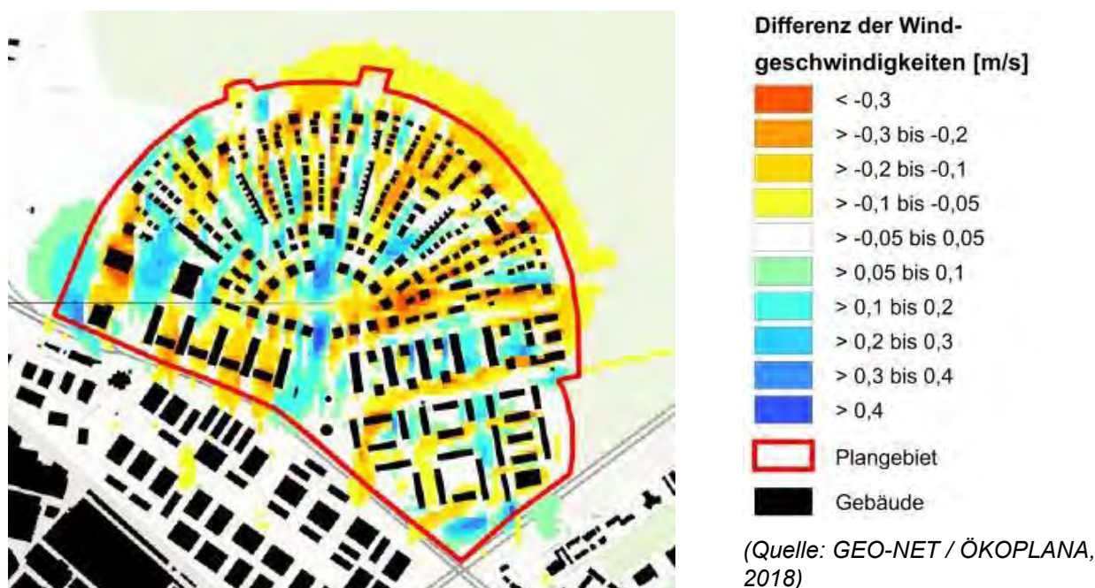
Abb. 28: Differenz der Windgeschwindigkeiten (m/s) im bodennahen Strömungsfeld um 4 Uhr morgens, 2 m über Grund zwischen Istzustand und Planzustand
