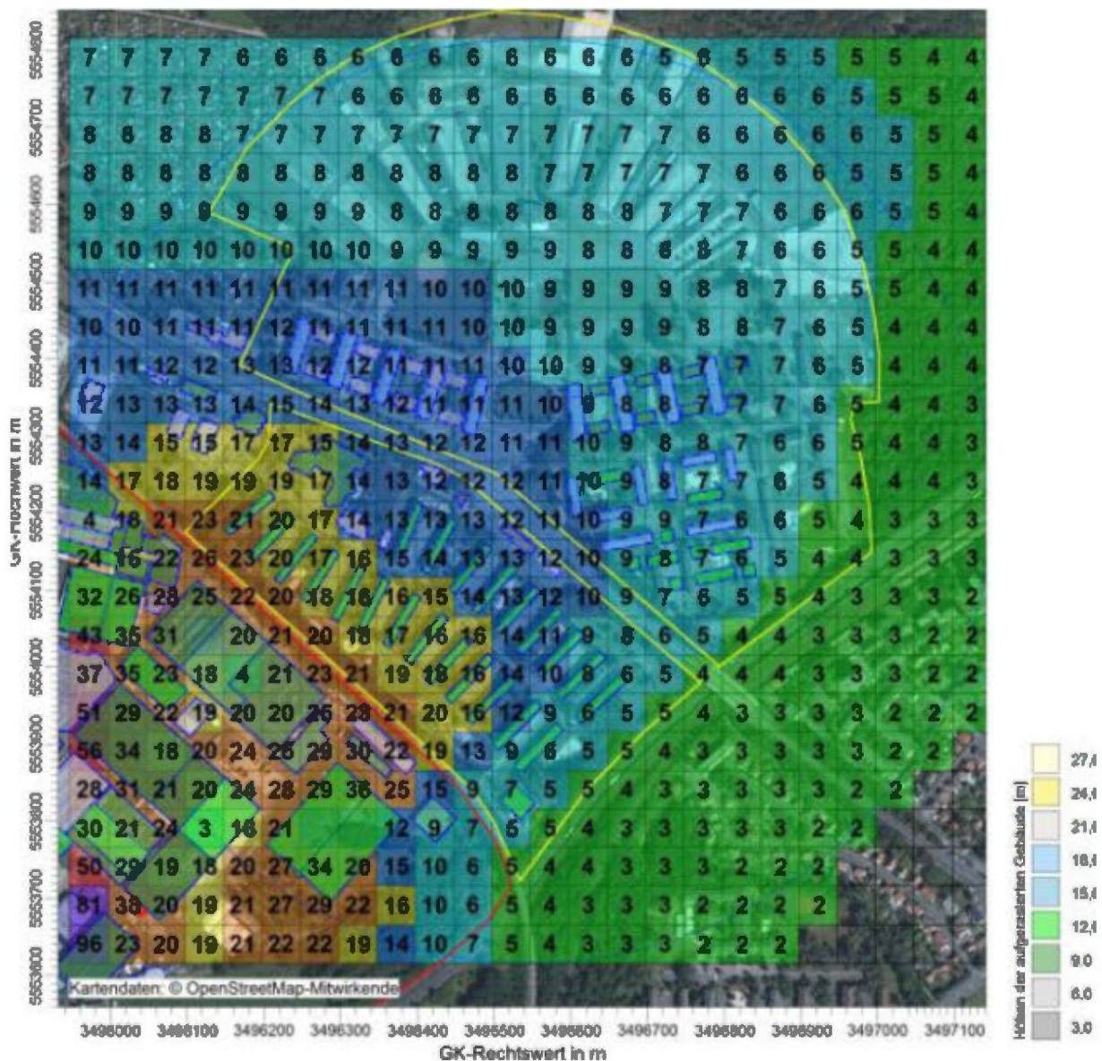
Abbildung 16: Ergebnis der Ausbreitungsrechnung nach Umsetzung aller vorgesehener Minderungsmaßnahmen: Relative Häufigkeit der Geruchsstunden, verursacht durch die Fa. Dunlop.
