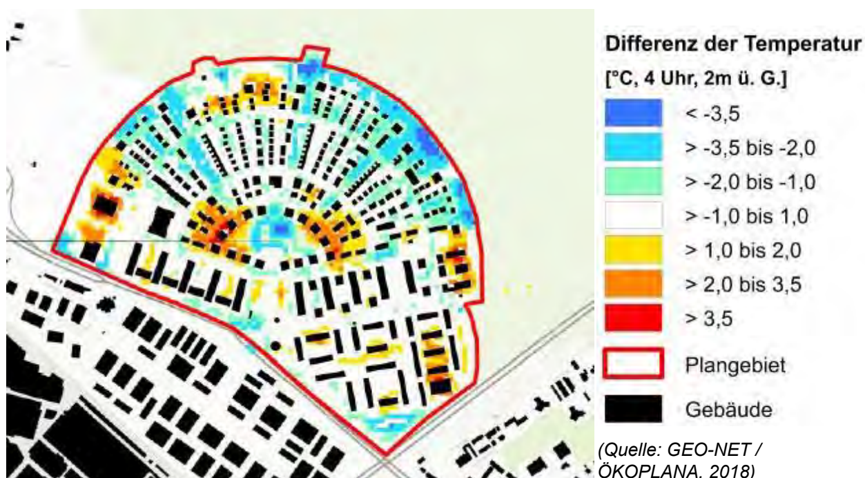
Abb. 27: Differenz der bodennahen Temperaturen (°C) um 4 Uhr morgens zwischen Istzustand und Planzustand
