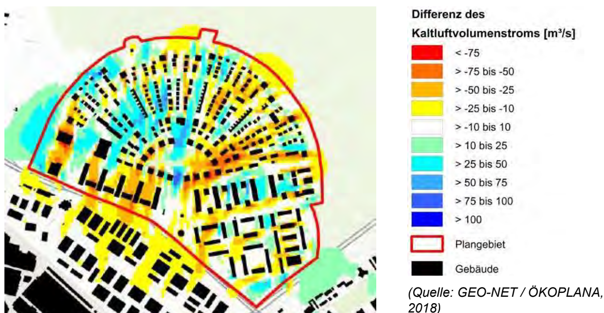
Abb. 29: Relative Änderung des Kaltluftstroms (m 3 /s) zwischen Istzustand und Planzustand
