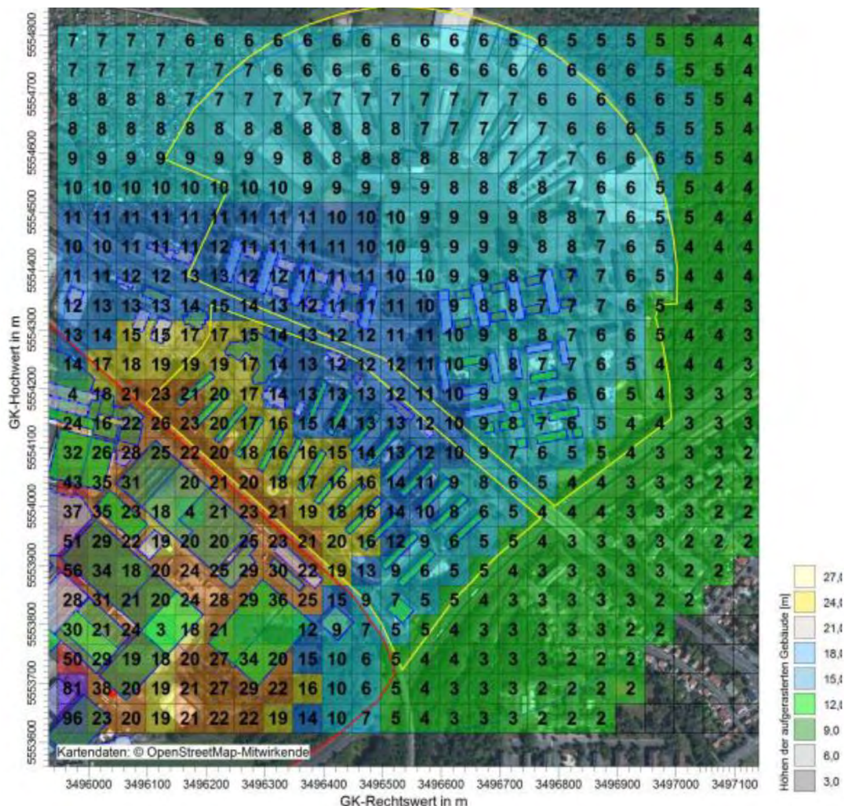
Abb. 36: Ergebnis der Ausbreitungsrechnung nach Umsetzung aller Minderungsmaßnahmen und unter Einbezug des Sicherheitszuschlags (Relative Häufigkeit der Geruchsstunden, verursacht durch die Fa. Dunlop)
