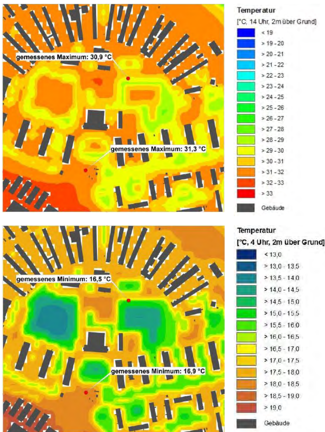
Abb. 19: Temperaturdifferenz in der bodennahen Luftschicht (2 m über Grund) zwischen Tag (14 Uhr oben) und Nacht (4 Uhr unten) Bodennahes Temperaturfeld (°C) (14 Uhr)
